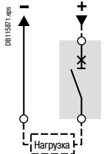
Выбор 1: стационарный 1-полюсный аппарат Compact NSX160N DC
