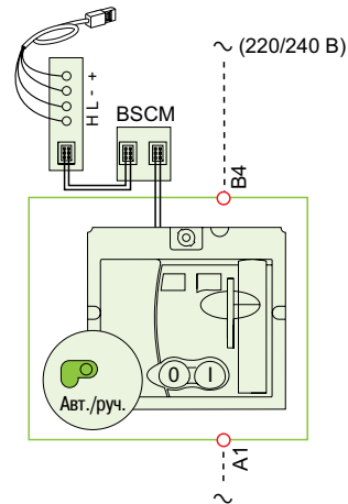
Коммутиционный мотор-редуктор (МТс) (1)
