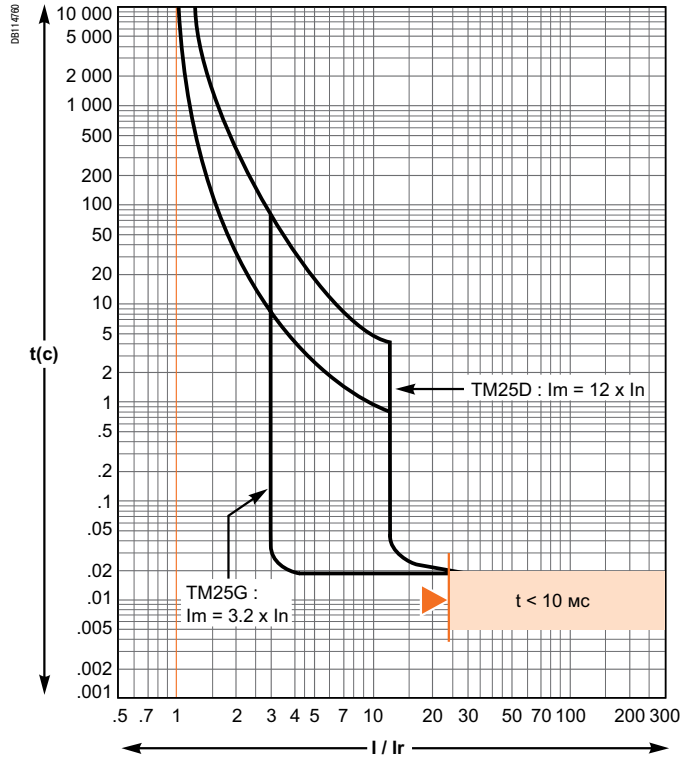
TM25D / TM25G
