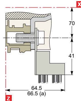
NSX100 - 250
