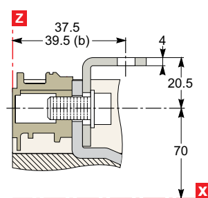
NSX100 - 250
