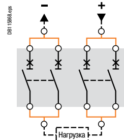
Выбор 2: 4-полюсный Compact NSX160 DC с параллельно-последовательным подключением 2 x 2 полюса
