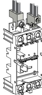
Цоколь аппарата 400/630 A
